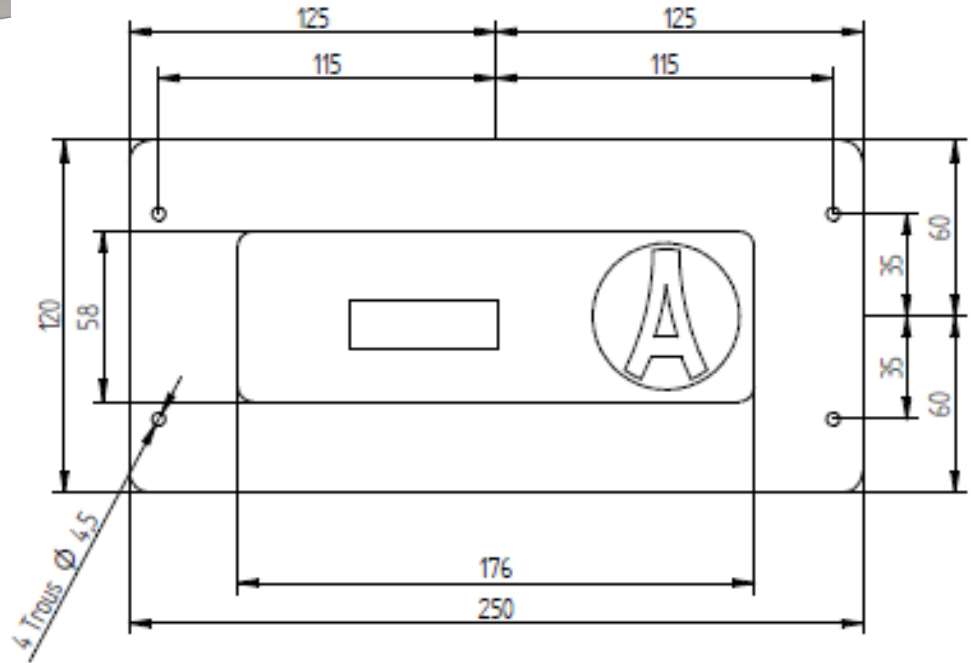
Dimension verre bandeau de commande
