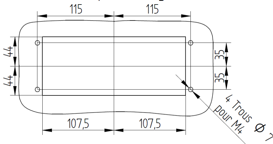
Dimensions de découpe 215x88mm
